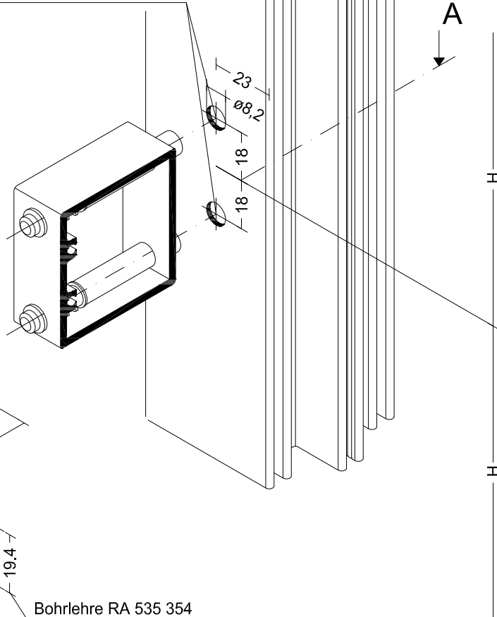
für Riegelverbinder RA 95 7101 und RA 95 7111
