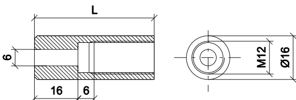
Sonnenschutzbolzen TYP A, L= 40 mm - 76 mm
