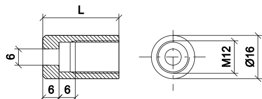
Sonnenschutzbolzen TYP B, L= 24 mm - 36 mm
