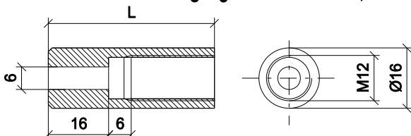
Sonnenschutzbefestigung 40 mm - 76 mm, TYP A
