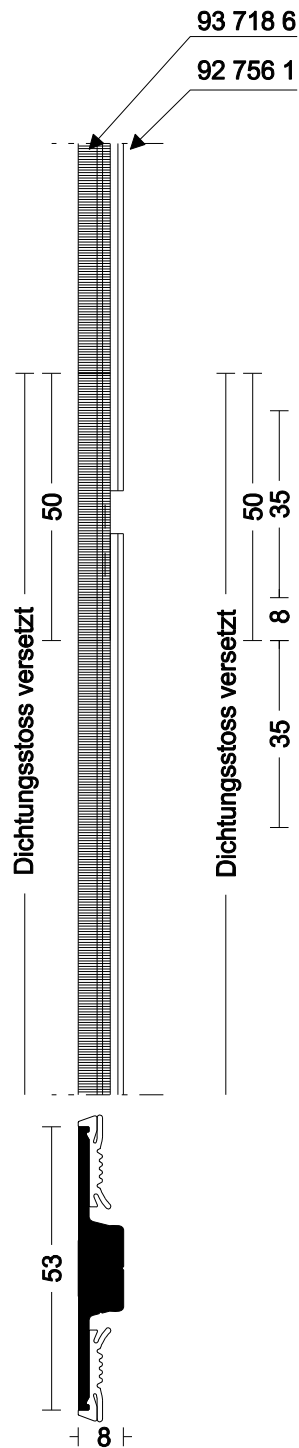
Vertikalstoss SG-Andruckprofil mit überlappender Dichtung
